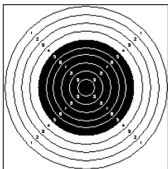
Standard 10 m löpande target; ISSF reglemente Sektion 6.3.2.7.2; diameter 50,5mm; svart riktprick från ring 5 till 10
