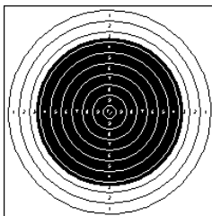
A10 50 m precisionstavlva gevär; ISSF reglemente Sektion 6.3.2.2; diameter 154,4mm; svart riktprick från del av ring 3 till ring 10, diameter 112,4mm
