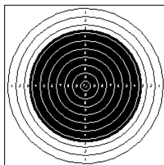
50m 50 m precisionstavla gevär; ISSF reglemente Sektion 6.3.2.2; diameter 154,4mm; svart riktprick från del av ring 3 till ring 10, diameter 112,4mm
