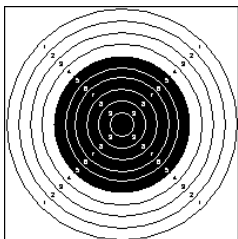
Final 10 m löpande target; ISSF reglemente Sektion 6.3.2.7.2; diameter 50,5mm; svart riktprick från ring 5 till 10
